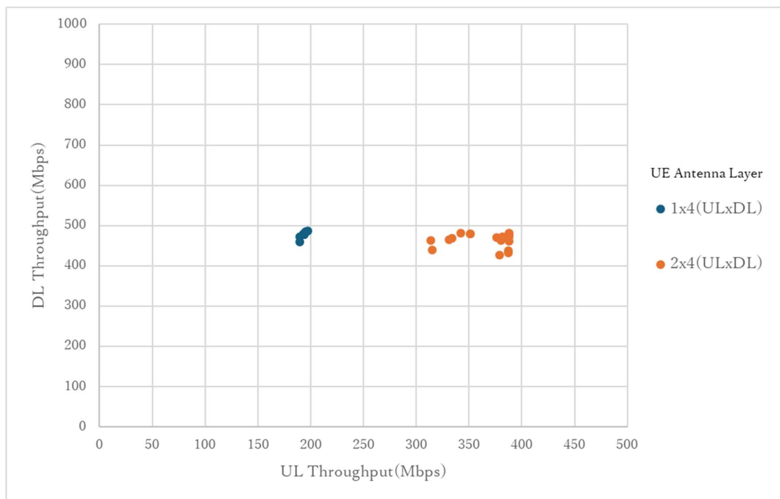
図 3-20 準同期 TCP スループット試験結果(グループ 2)
