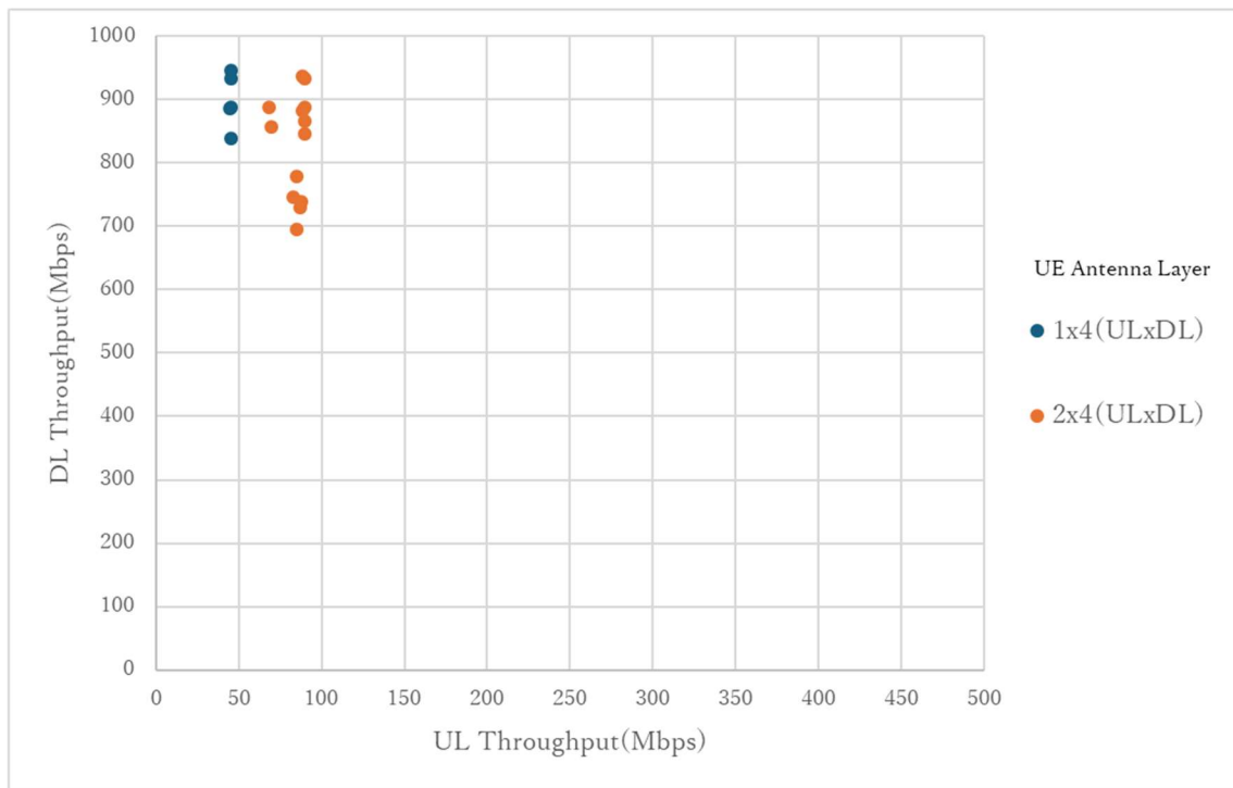
図 3-23 同期 TCP スループット試験結果(グループ 3)
