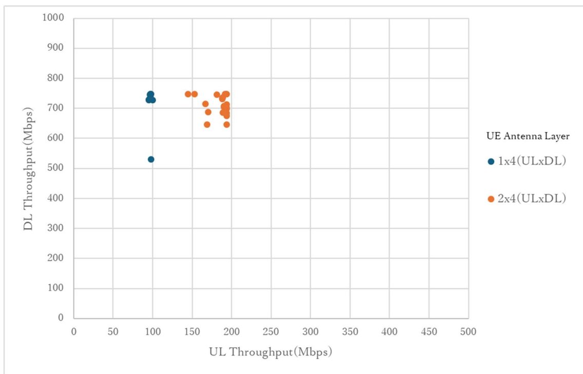
図 3-19 同期 TCP スループット試験結果(グループ 2)
