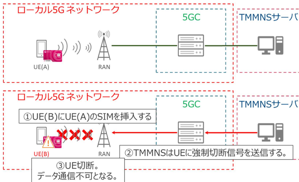
図 4-3 SIM スワップ防御テストシナリオ
