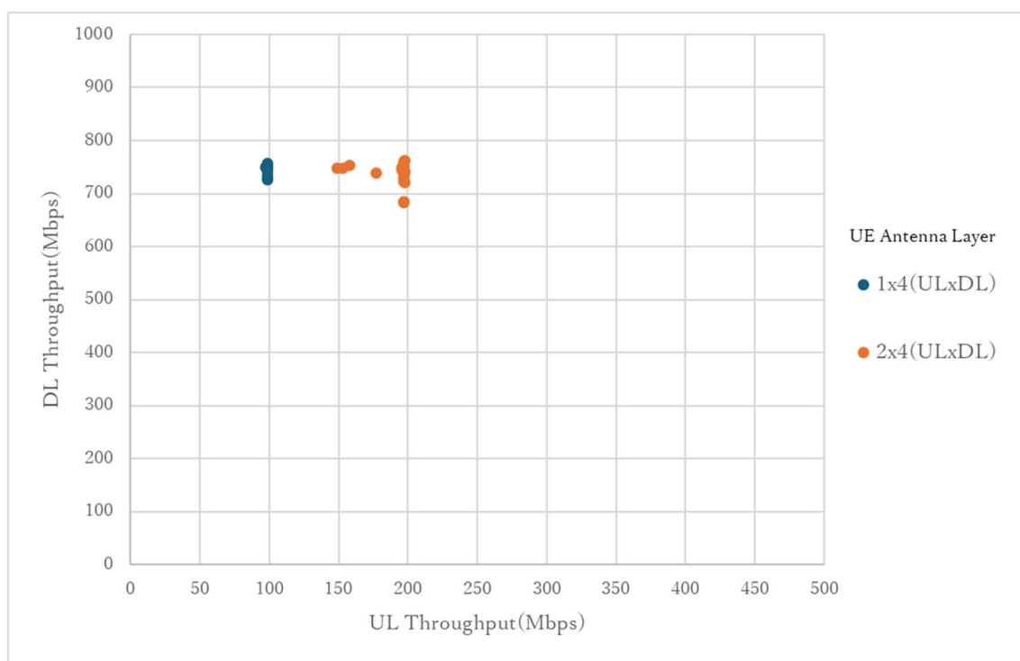
図 3-17 同期 UDP スループット試験結果(グループ 2)
