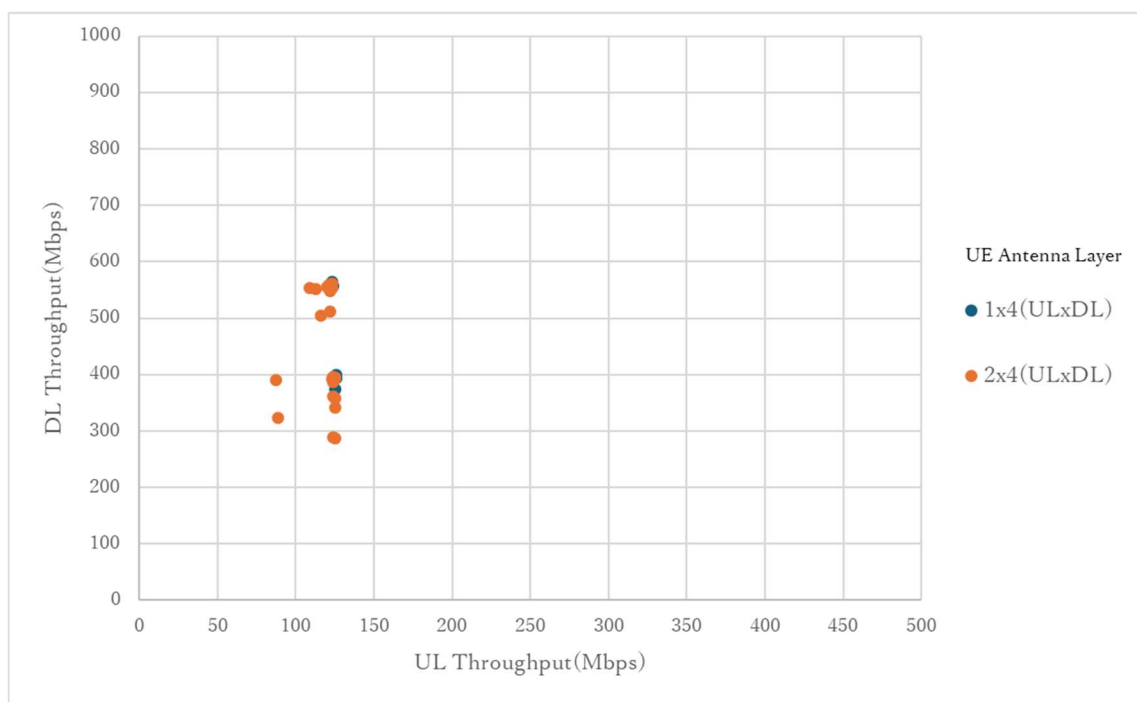
図 3-16 準同期 TCP スループット試験結果(グループ 1)
