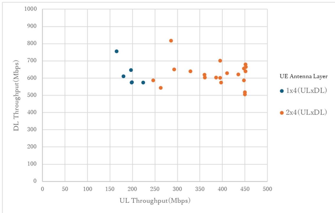
図 3-30 準同期 UDP スループット試験結果(グループ 5)
