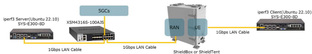
図 3-11 スループット試験構成
