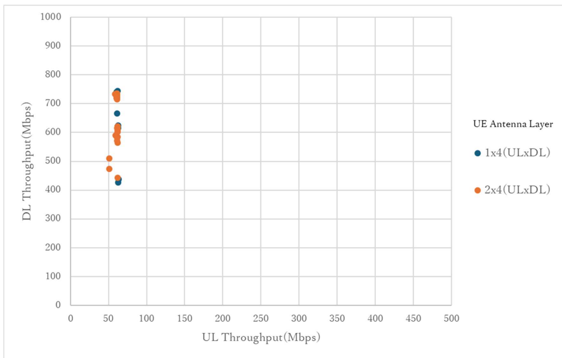
図 3-15 同期 TCP スループット試験結果(グループ 1)
