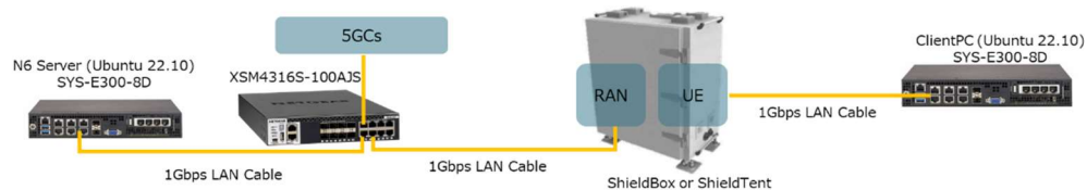
図 3-1 相互接続試験構成
