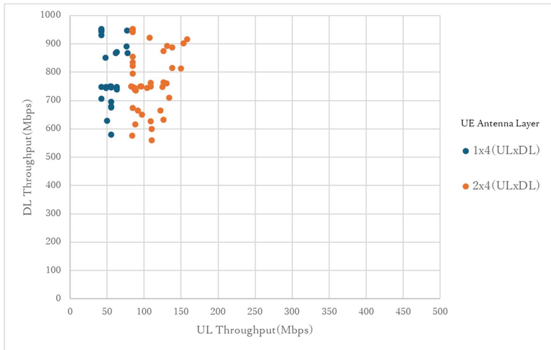
図 3-25 同期 UDP スループット試験結果(グループ 4)
