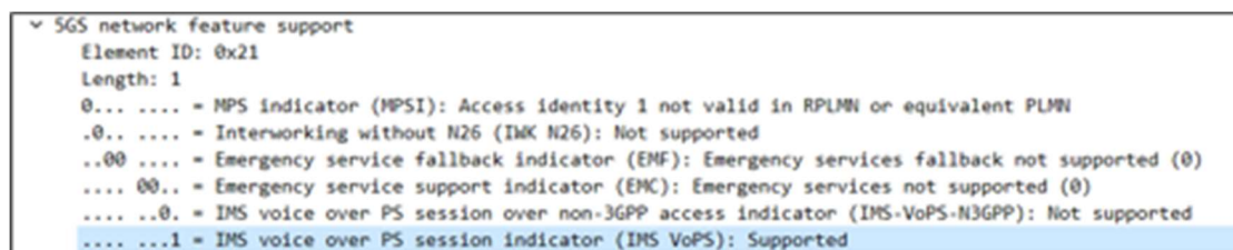
図 3-7 IMS_VoPS をサポートする 5GC の NGAP_Registration Accept 信号例
