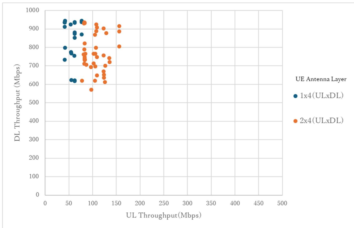
図 3-27 同期 TCP スループット試験結果(グループ 4)
