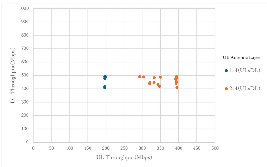
図 3-18 準同期 UDP スループット試験結果(グループ 2)
