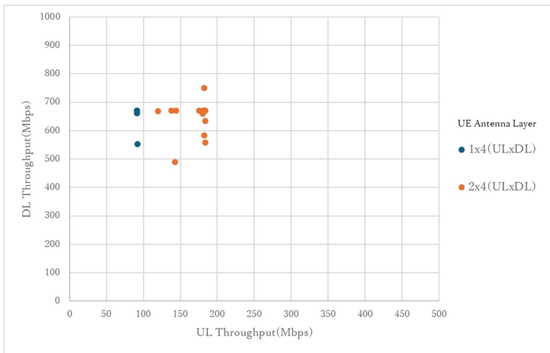
図 3-22 準同期 UDP スループット試験結果(グループ 3)
