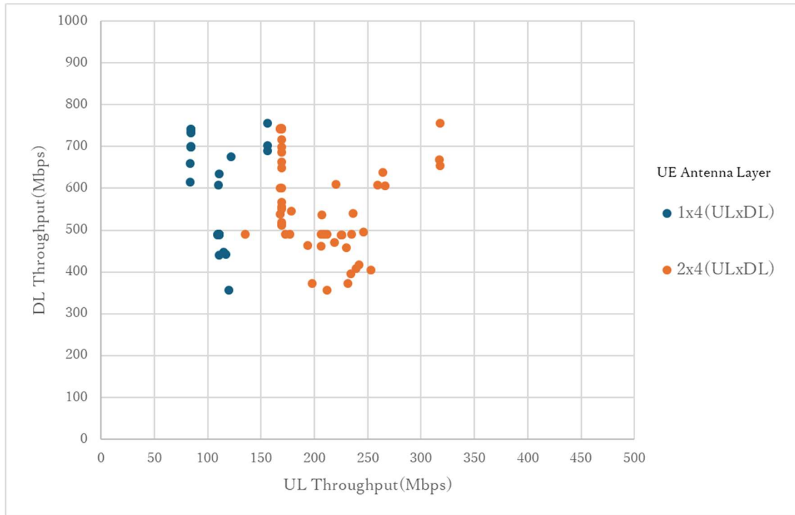
図 3-26 準同期 UDP スループット試験結果(グループ 4)
