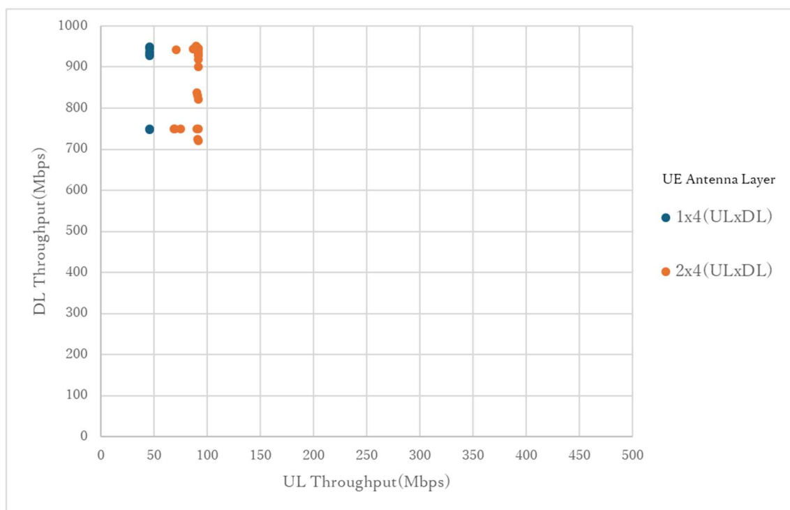
図 3-21 同期 UDP スループット試験結果(グループ 3)
