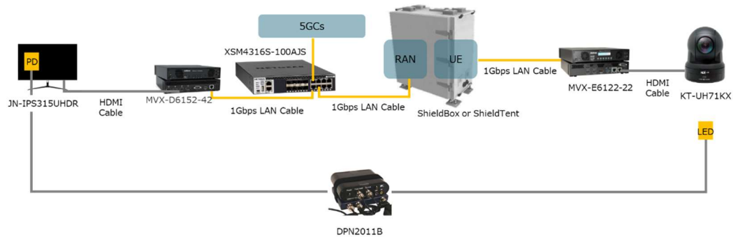
図 3-33 4K 動画伝送遅延試験構成
