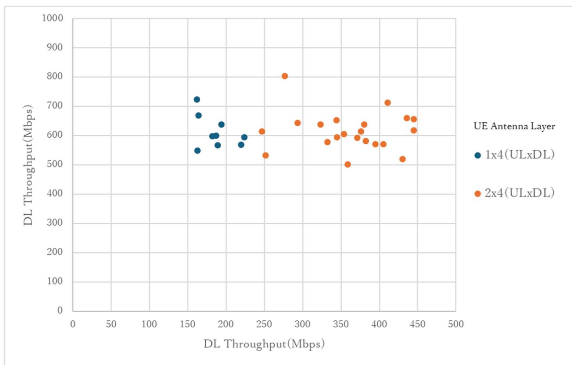
図 3-32 準同期 TCP スループット試験結果(グループ 5)
