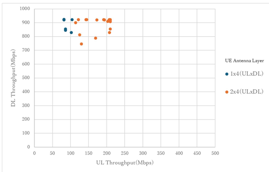
図 3-29 同期 UDP スループット試験結果(グループ 5)
