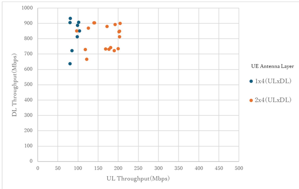
図 3-31 同期 TCP スループット試験結果(グループ 5)
