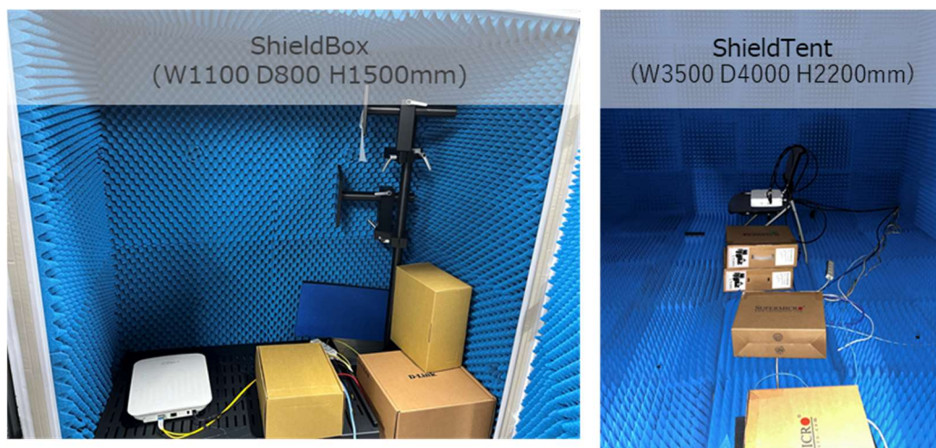
図 3-2 シールドボックスおよびシールドテント
