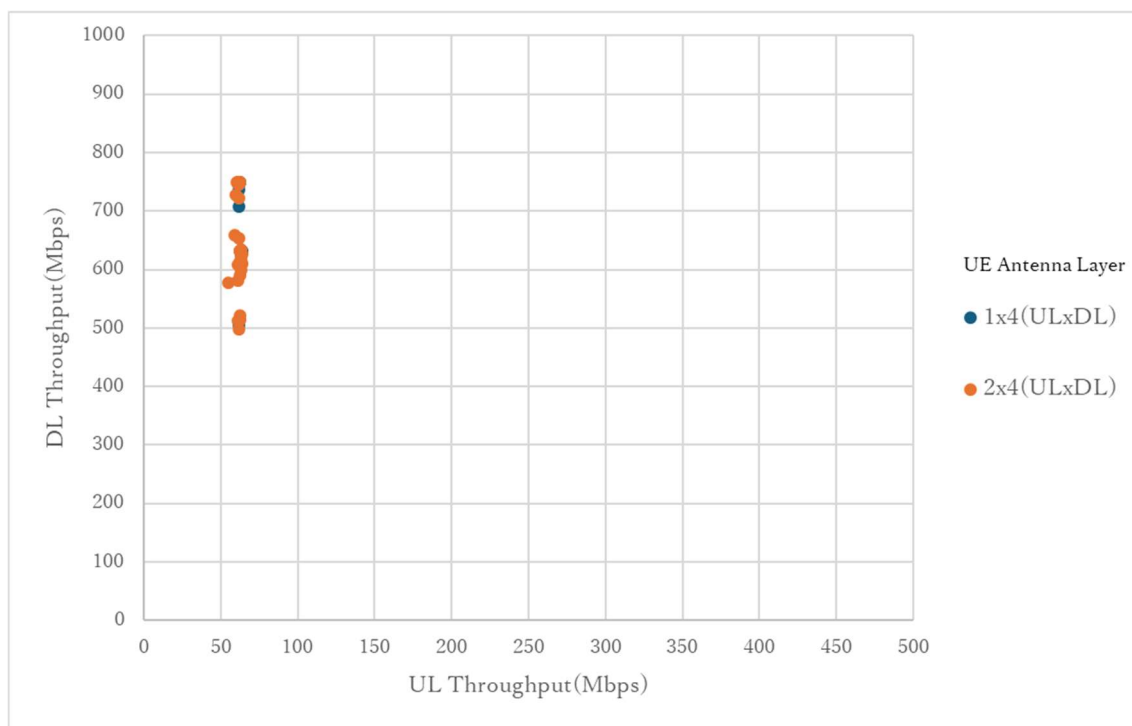
図 3-13 同期 UDP スループット試験結果(グループ 1)
