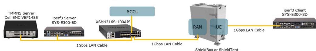
図 4-1 セキュリティ試験構成
