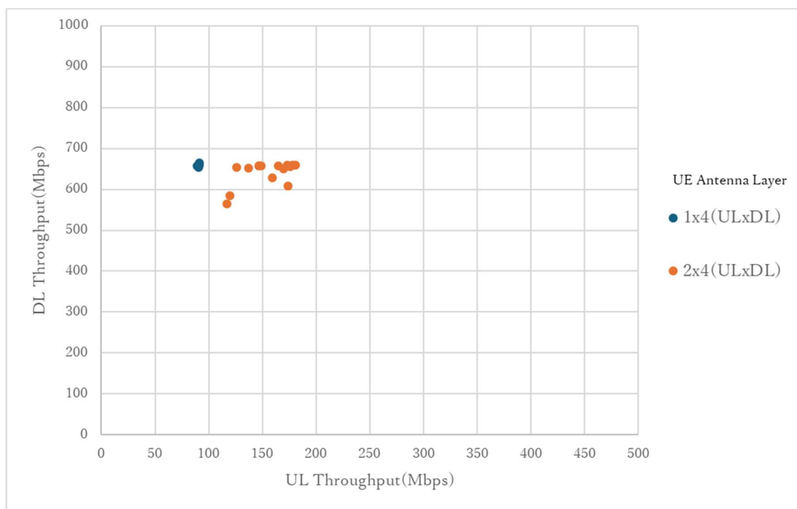
図 3-24 準同期 TCP スループット試験結果(グループ 3)
