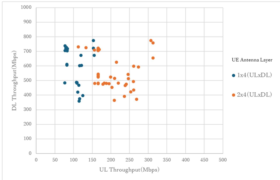
図 3-28 準同期 TCP スループット試験結果(グループ 4)
