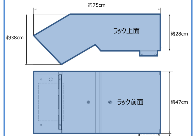
②ラックの寸法
