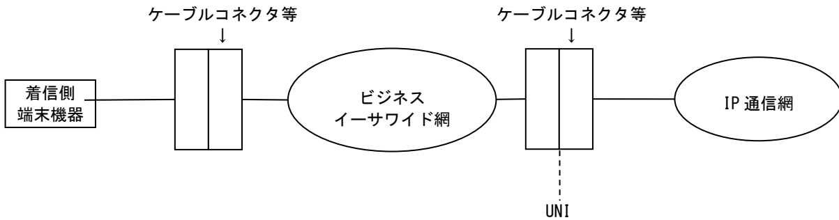
図 1-8 ビジネスイーサワイド接続タイプのインターフェース規定点
