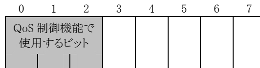
図 4-2 ToS フィールドの構成
