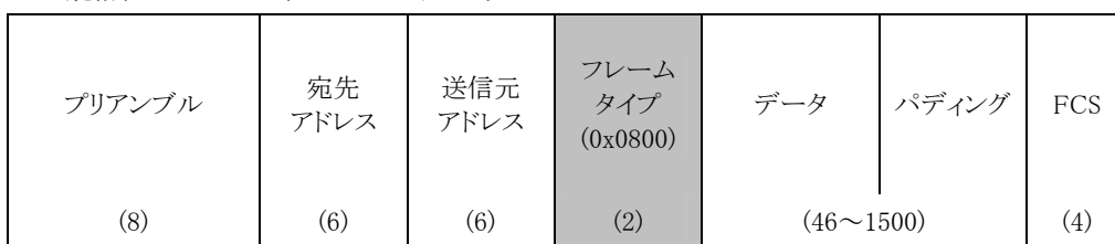
DIX 規格(Ethernet ver.2)フレームフォーマット
