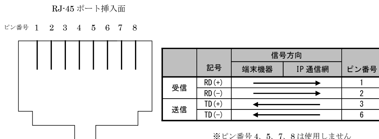
図 13-1 挿入面から見た RJ-45 ポートのピン配置
