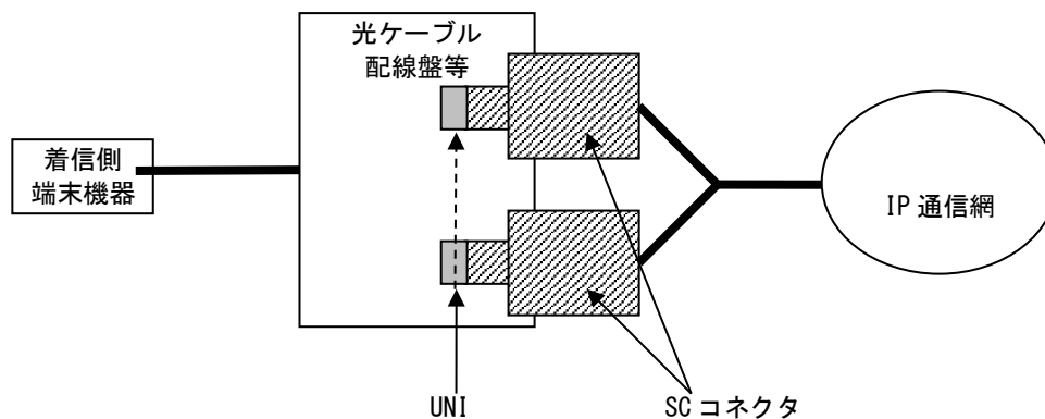
図 12-5 GigabitEthernet/10 GigabitEthernet タイプのインタフェース規定点
