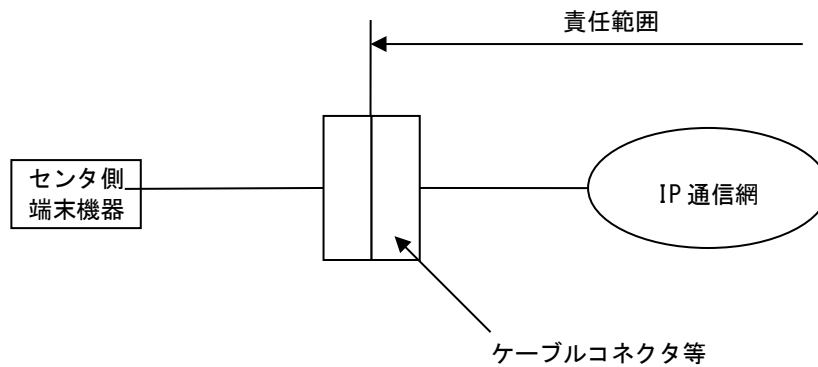
図 19-5 フレッツ・キャストにおける施工・保守上の責任範囲
