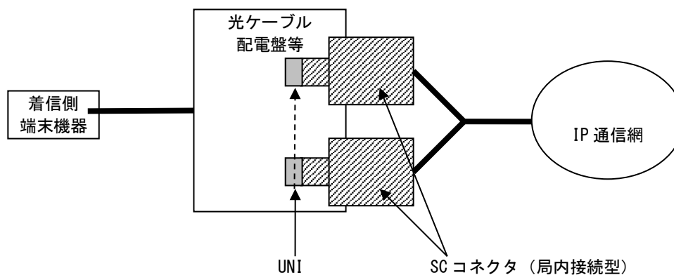
図 12-3 Ethernet/FastEthernetタイプのインタフェース規定点
