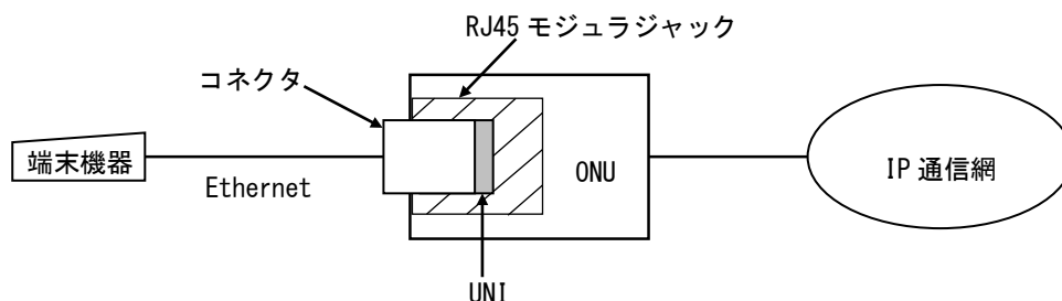
図 8-3 インタフェース規定点
