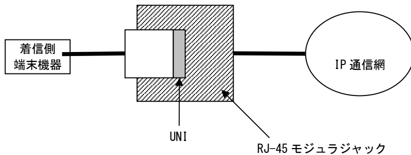
図 17-4 100Mb/sメニューのインタフェース規定点
