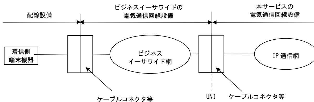
図 17-13 ビジネスイーサワイド接続タイプの分界点
