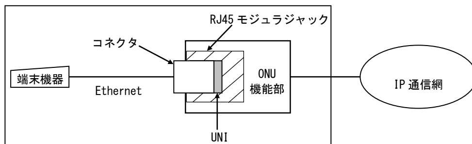
図 11-1 インタフェース規定点
