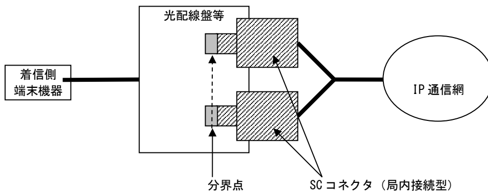
図 12-10 FastEthernetタイプにおける施工・保守上の責任範囲分界点
