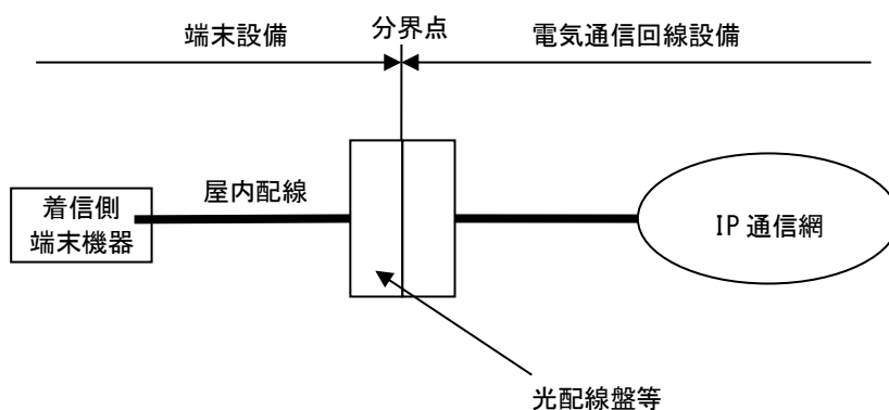
図 12-7 GigabitEthernet/10 GigabitEthernetタイプの分界点
