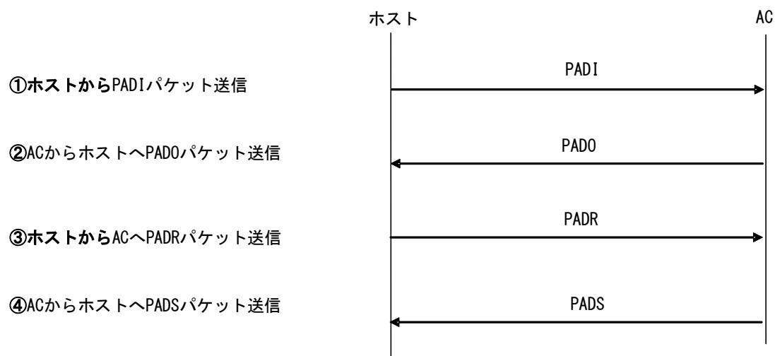
図 10-1 PPPoE セッション確立手順
