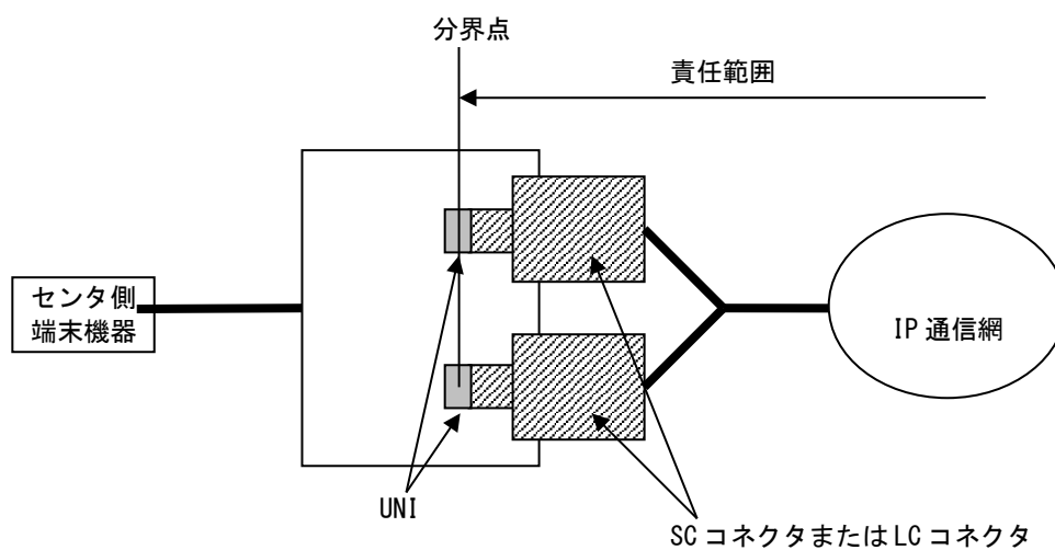
図 19-6 フレッツ・キャストにおける施工・保守上の責任範囲分界点
