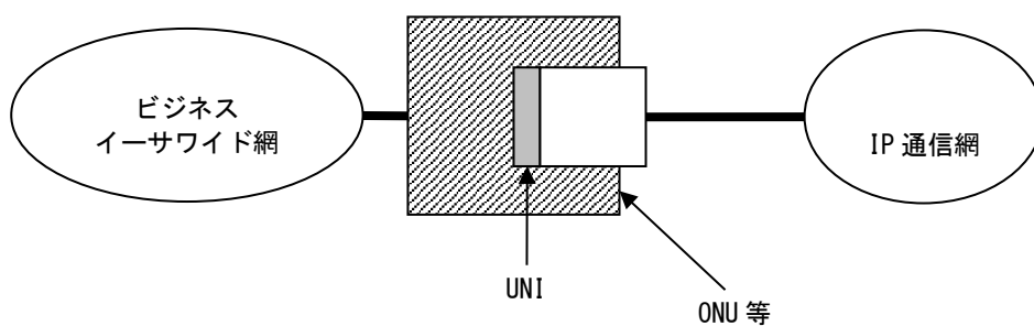
図 17-10 100Mb/sメニューのインタフェース規定点
