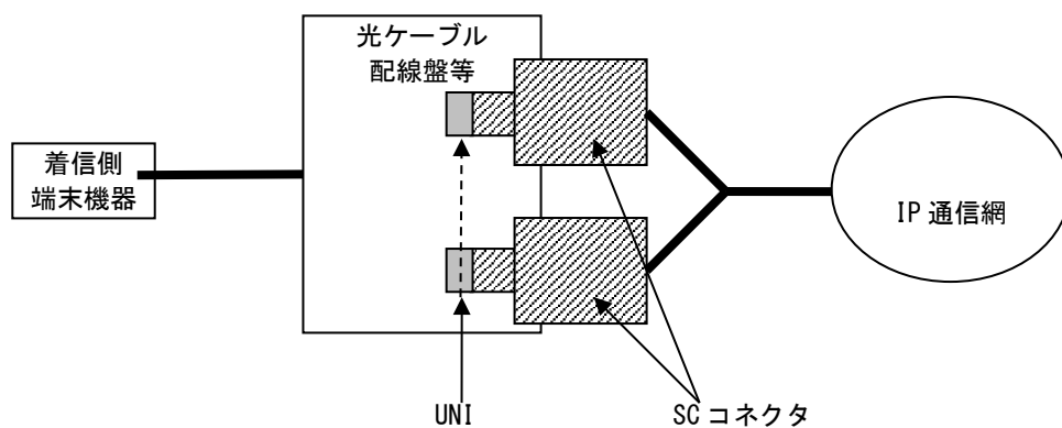
図 17-5 100Mb/sメニューのインタフェース規定点
