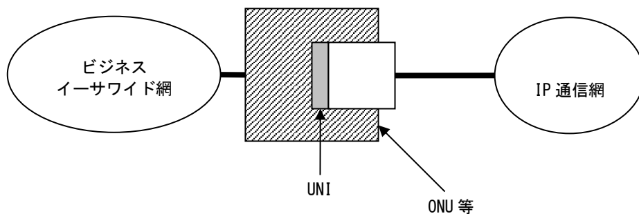
図 17-9 10Mb/sメニューにおけるインタフェース規定点
