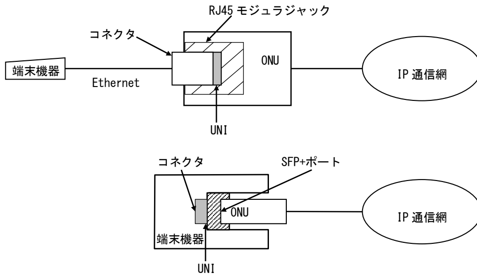
図 4-3 フレッツ 光ネクストのインタフェース規定点
