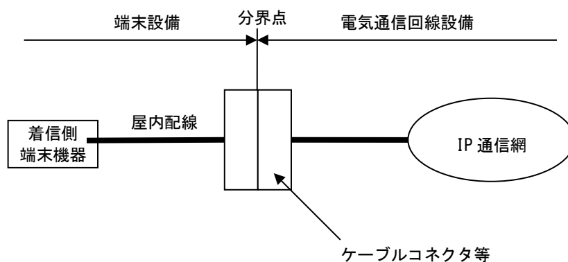
図 17-11 局内接続タイプの分界点
