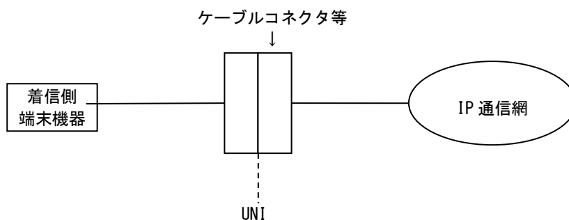
図 17-2 局内接続タイプのインタフェース規定点
