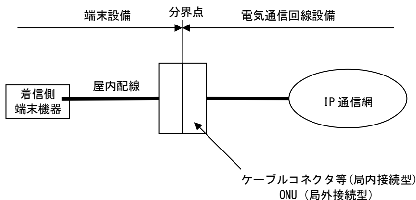
図 12-6 Ethernet/FastEthernetタイプの分界点
