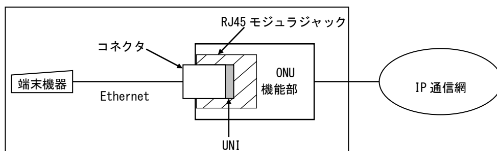
図 7-1 フレッツ 光ネクストのインタフェース規定点
