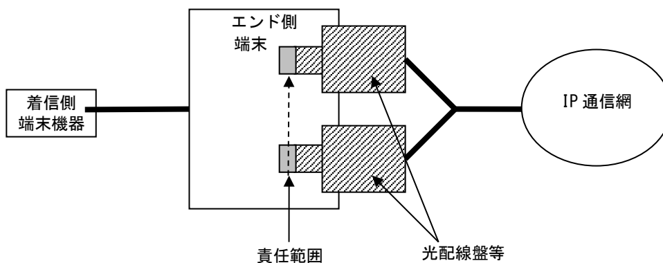
図 12-14 GigabitEthernet/10 GigabitEthernetタイプにおける施工・保守上の責任範囲分界点
