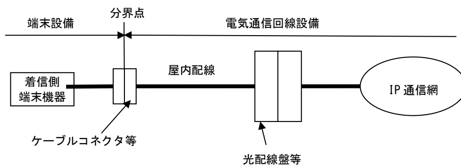
図 17-12 収容エリア内接続タイプの分界点
