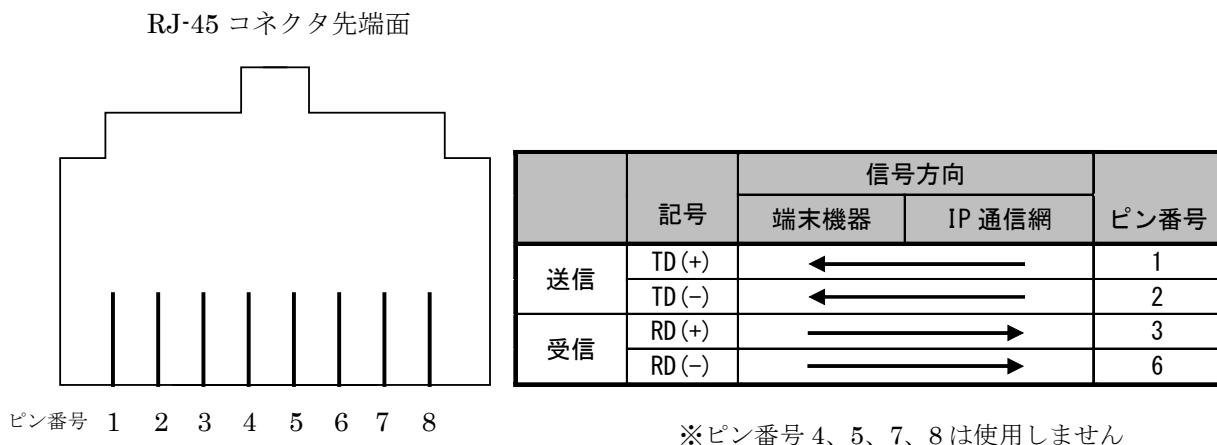
図 18-2 コネクタ先端面から見た RJ-45 コネクタのピン配置
