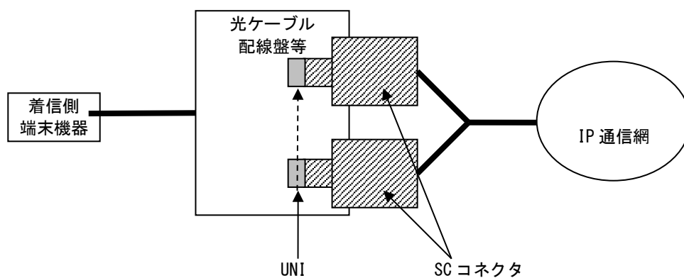
図 17-7 100Mb/sメニューのインタフェース規定点
