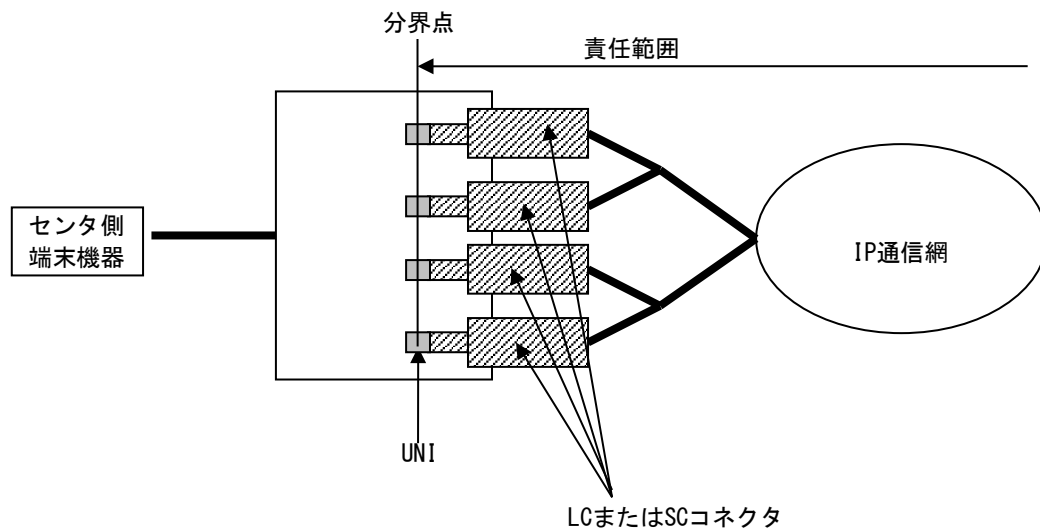
図 23-7 本サービスにおける施工・保守上の責任範囲分界点
