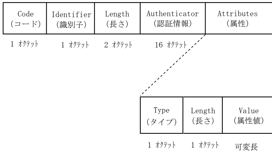
図 16-1 認証関連通信パケットのパケットフォーマット
