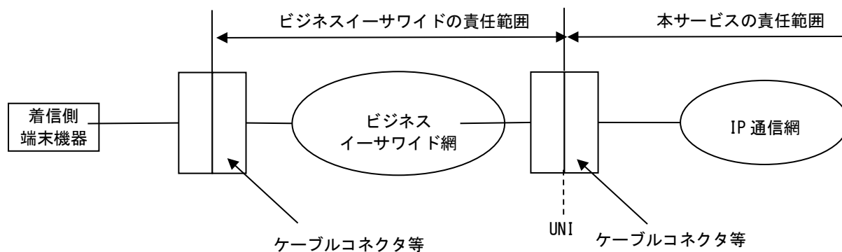
図 17-16 ビジネスイーサワイド接続タイプの施工・保守上の責任範囲
