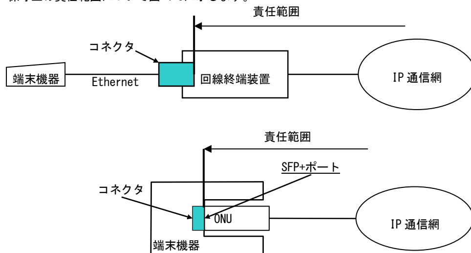
図 4-5 施工・保守上の責任範囲
