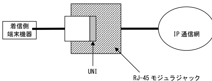
図 17-3 10Mb/sメニューのインタフェース規定点
