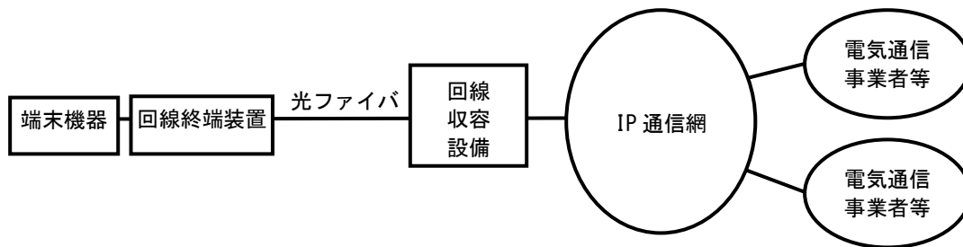
図 4-1 フレッツ 光ネクストの基本構成
