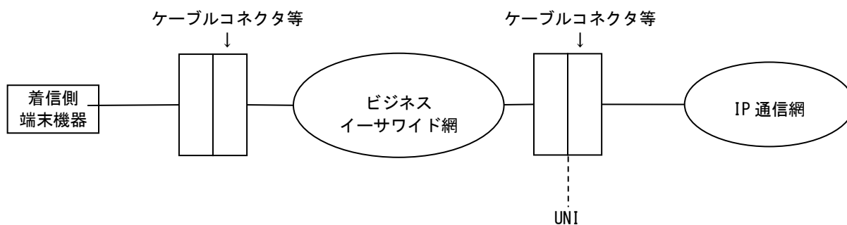
図 17-8 ビジネスイーサワイド接続タイプのインタフェース規定点
