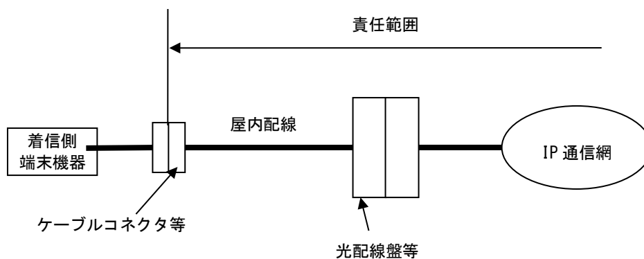
図 12-13 GigabitEthernet/10 GigabitEthernetタイプにおける施工・保守上の責任範囲
