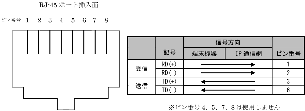
図 18-1 挿入面から見た RJ-45 ポートのピン配置
