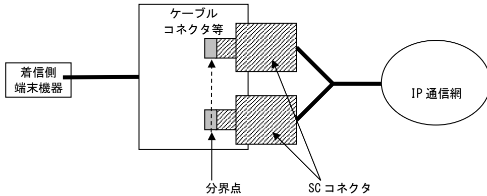
図 12-12 GigabitEthernet/10 GigabitEthernetタイプにおける施工・保守上の責任範囲分界点
