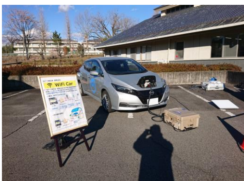
EV車の電源供給・衛星通信による Wi-Fi 提供
