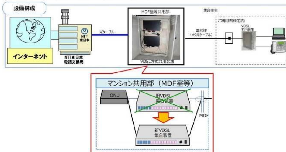
NTT東日本 集合住宅用装置 交換工事 イメージ図
