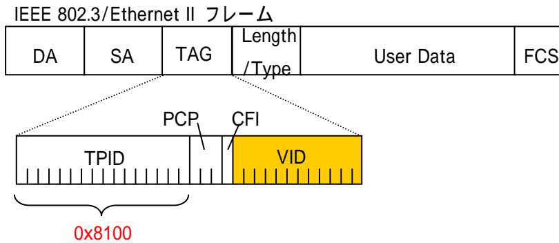
図 7-1-3 VID 識別子の位置
