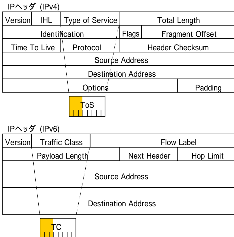
図 7-1-1 TOS/TC 識別子の位置
