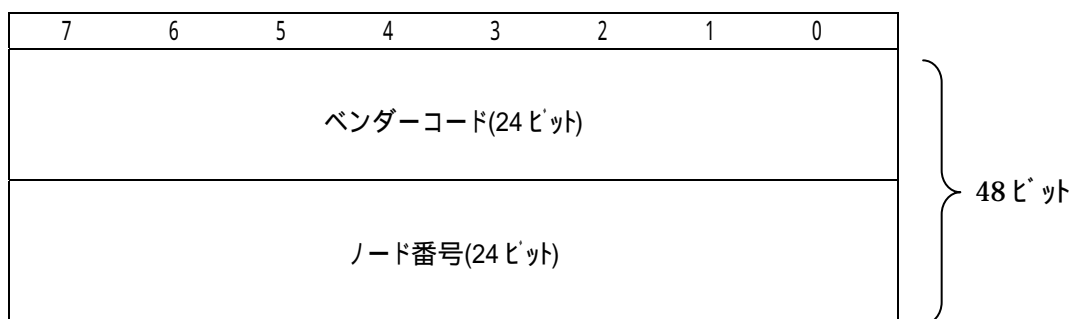
図 5-2-3 MAC アドレスの構成
