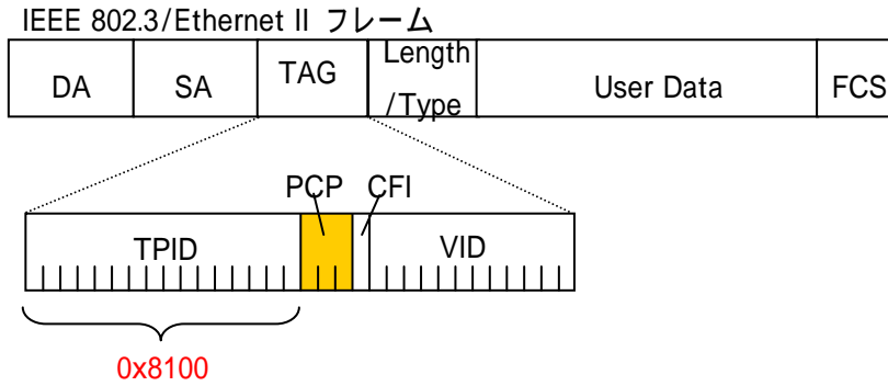
図 7-1-2 CoS 識別子の位置
