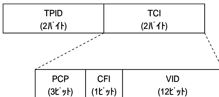
図 5-2-2b IEEE802.1Q の VLAN タグフォーマット
